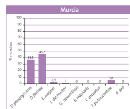
Tyrophagus putrescentiae
