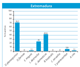
Dermatophagoides pteronyssinus
