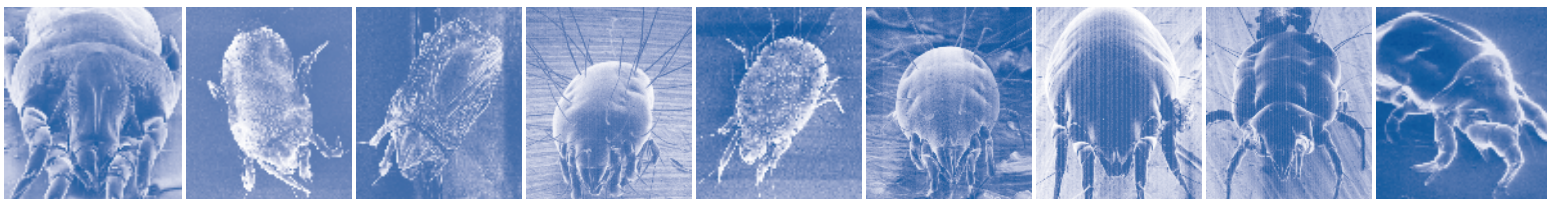
Dermatophagoides pteronyssinus
