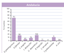
Euroglyphus maynei
